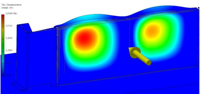
Desplazamiento máximo (Protección lateral)
