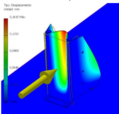
Desplazamiento máximo (Protección individual)
