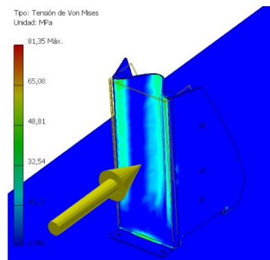
Tensión de deformación (Protección individual)
