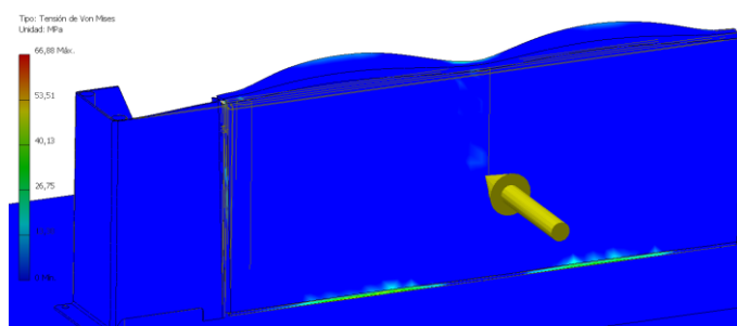
Tensión de deformación (Protección lateral)
